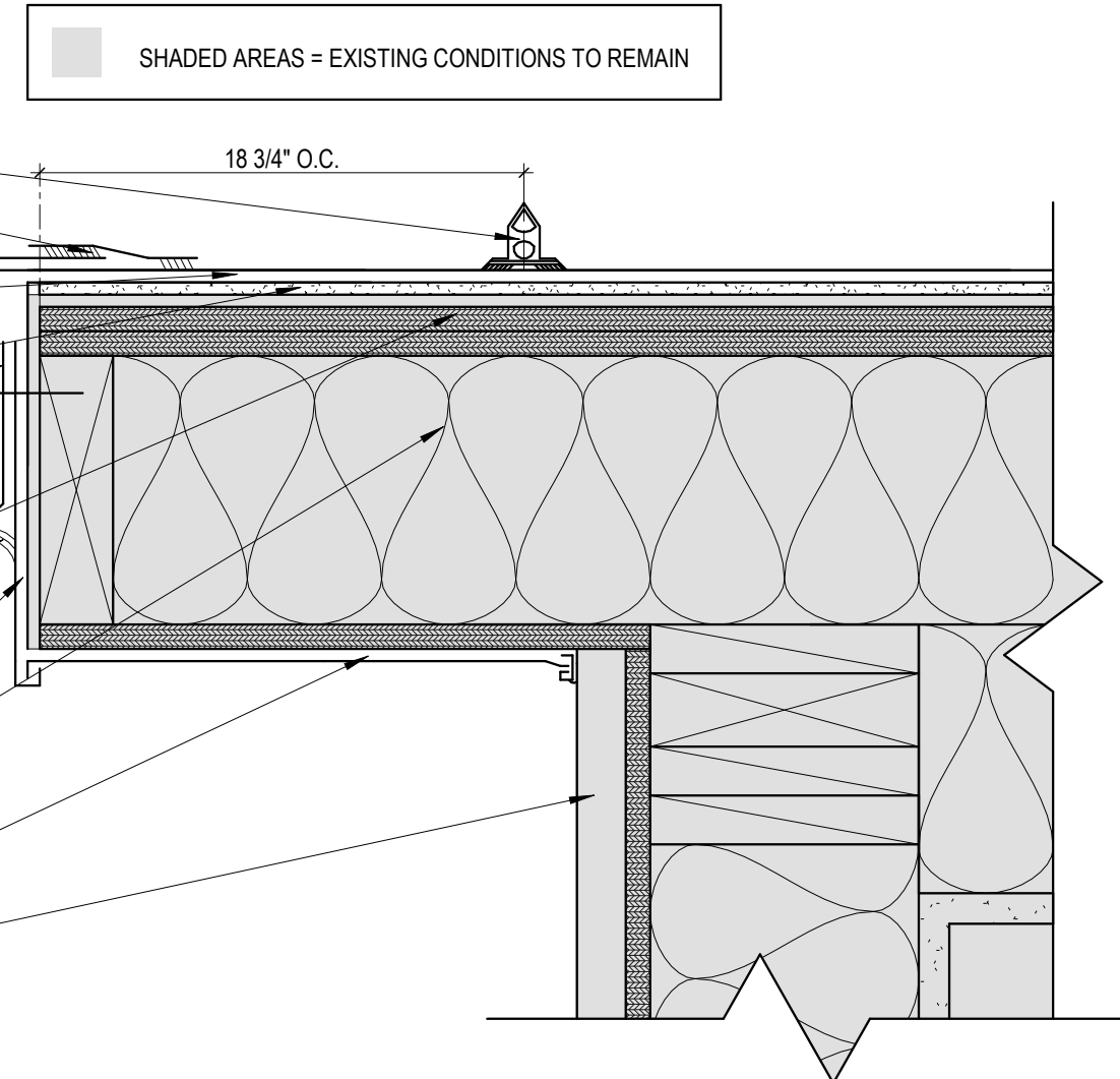
5 Fascia Detail Scale: 3\"/>
