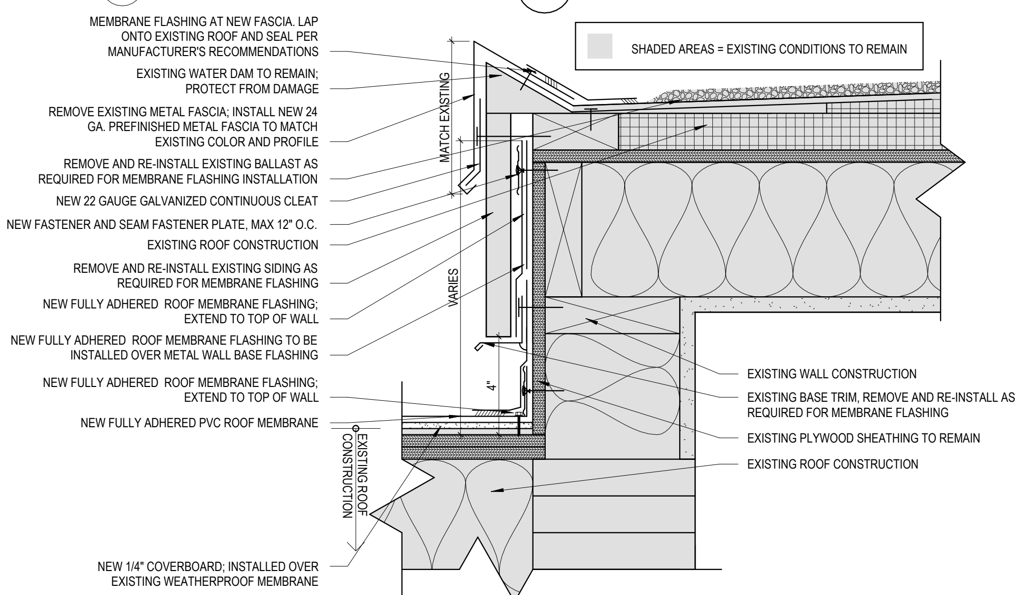
4 Fascia Detail Scale: 3\"/>
