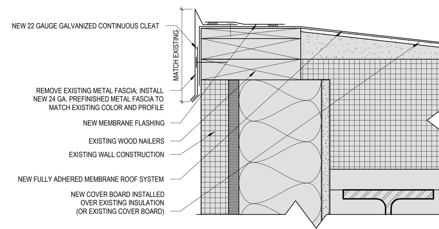
2 Roof Edge Detail Scale: 3" = 1'-0"
