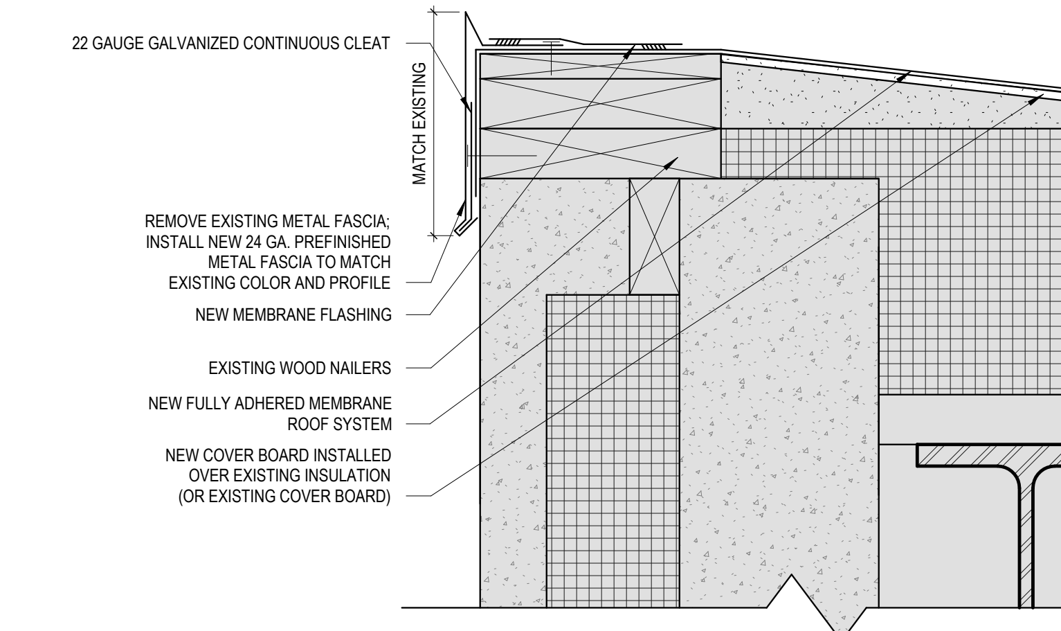
3 Roof Edge Detail Scale: 3" = 1'-0"
